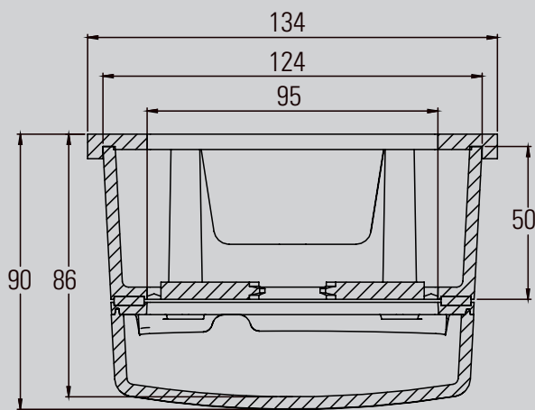
50 mm opbouwrand – boven aanzicht
