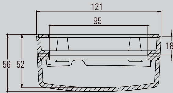
18 mm opbouwrand – boven aanzicht
