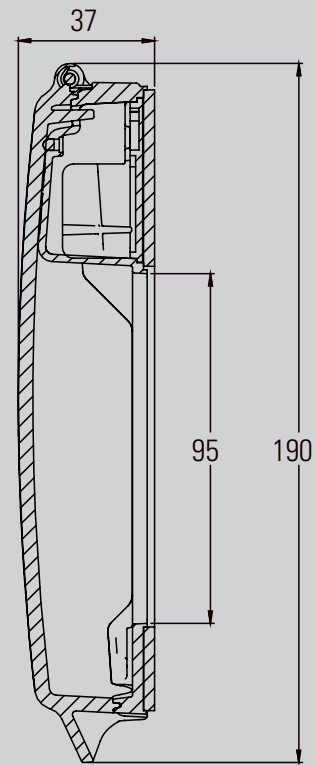
Inbouw model – zij aanzicht
