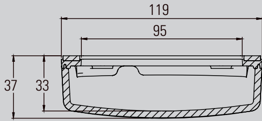
Inbouw model – boven aanzicht
