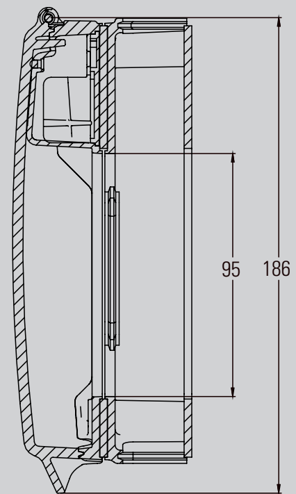
32mm opbouwrand – zij aanzicht
