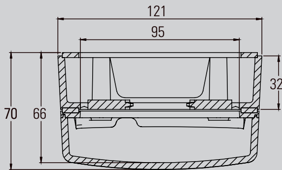
32 mm opbouwrand – boven aanzicht
